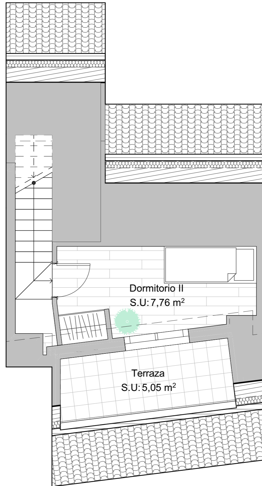
ENTREPLANTA
