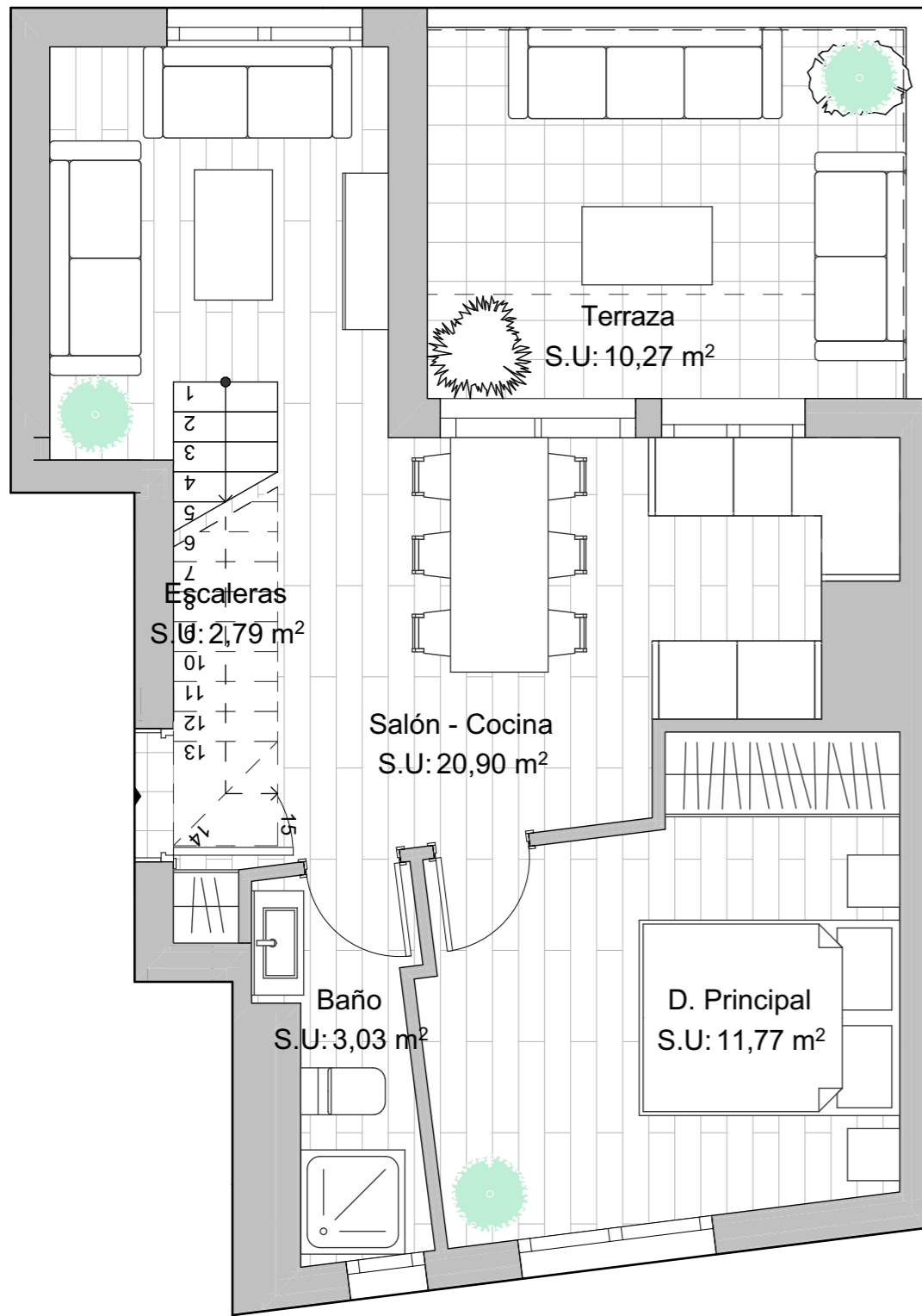
ÁTICO
