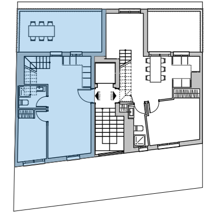
ÁTICO
