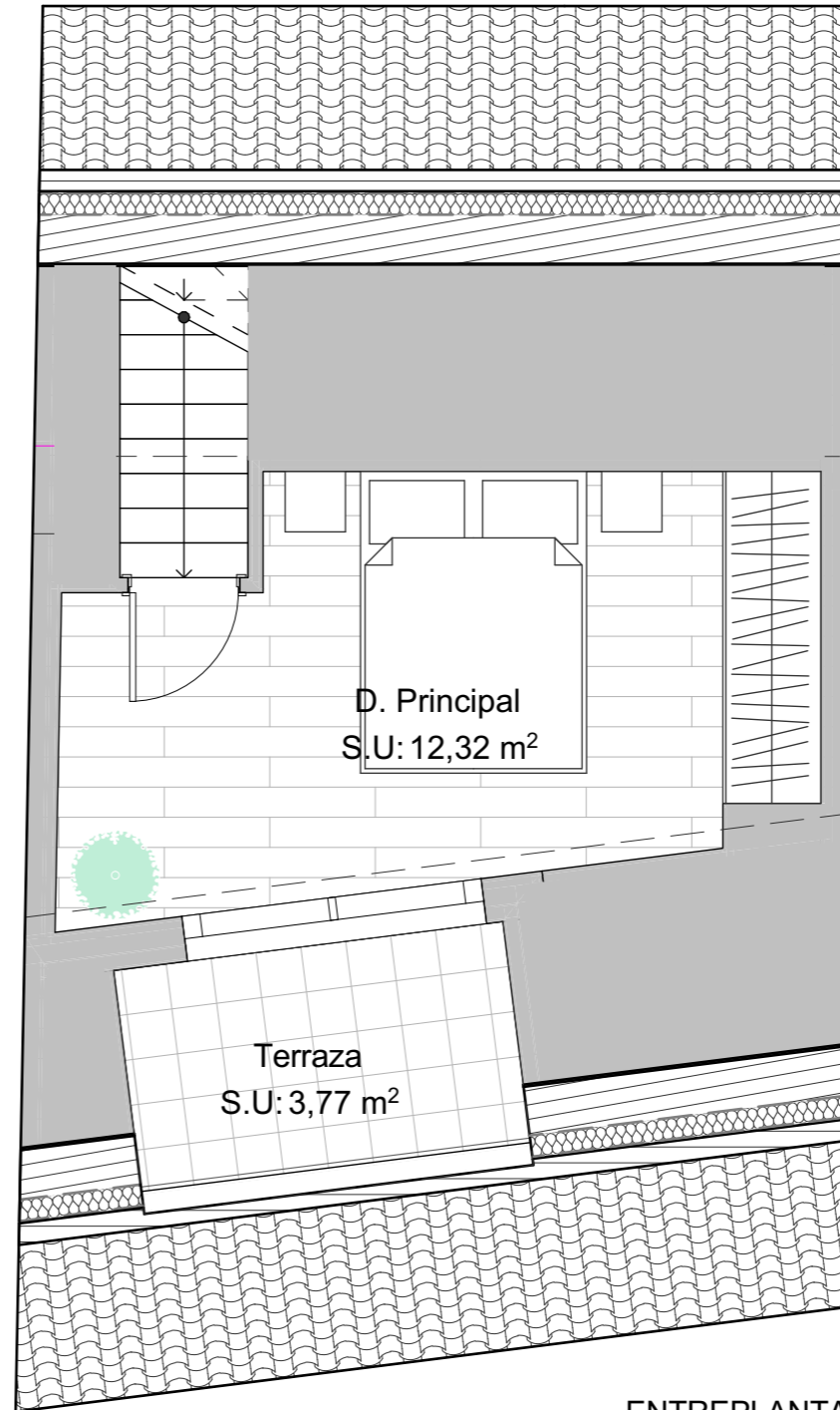
ENTREPLANTA
